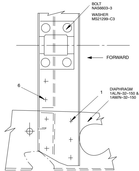
SECTION D-D
